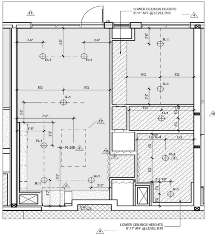
10 UNIT A5M4 RCP 4-118.2 Scale: 1/4" = 1'-0"
