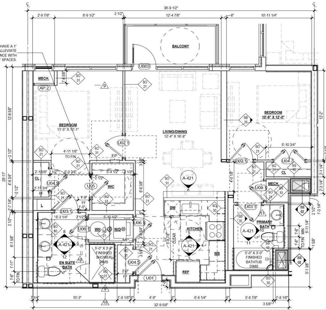
1 A-421 UNIT B1 PLAN Scale: 1/4" = 1'-0"
