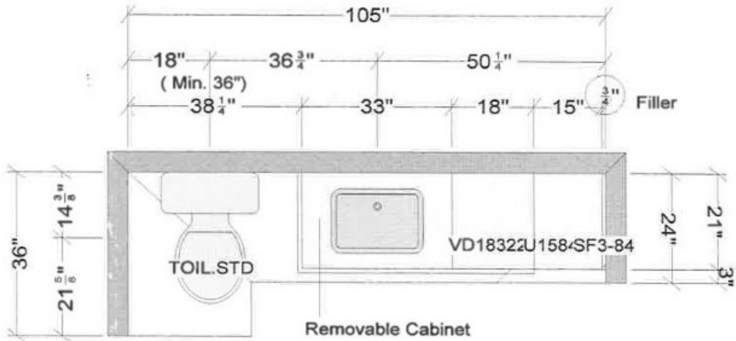
Unit B3 EN Suite Bath
