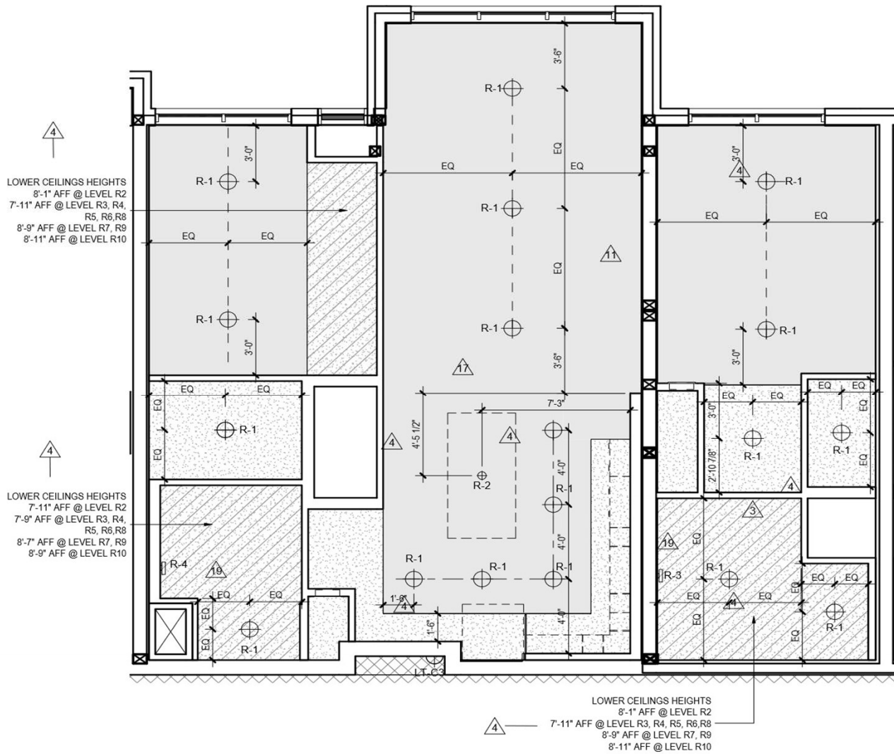
4 UNIT B3M1 RCP A-423 Scale: 1/4" = 1'-0"
